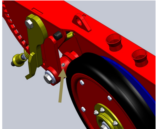
Kuva 5.4 Kylkipyörän varren nivelholkki.
