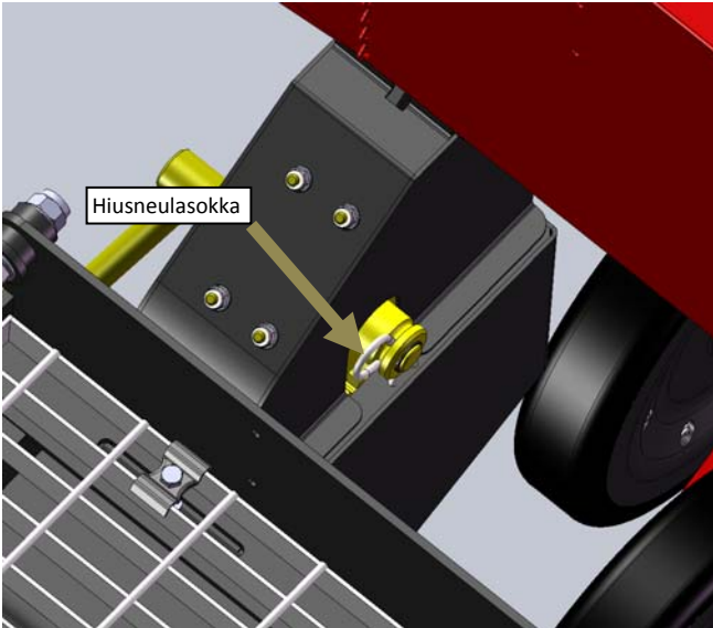
Kuva 3.3.1 Voimansiirron vapautus.
