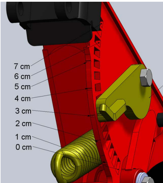
Kuva 3.2.2 Syvyydensäädön lovet.
