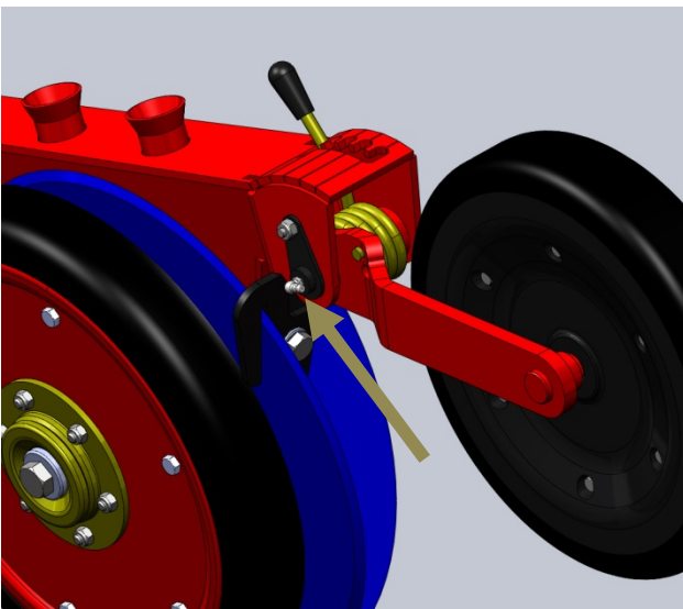
Kuva 5.5 Peittopyörän nivelholkki.
