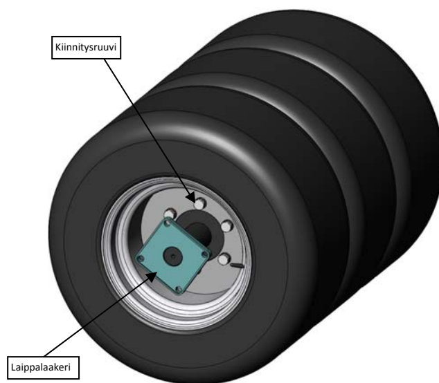
Kuva 5.14 Rengaspaketin purku.
