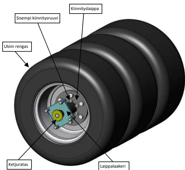
Kuva 5.13 Rengaspaketin (tässä=vasen) purku.
