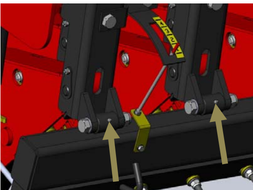
Kuva 5.7 Vannaspainoakseli.
