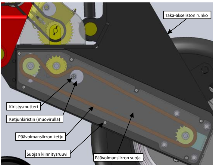
Kuva 5.1 Päävoimansiirron ketju.
