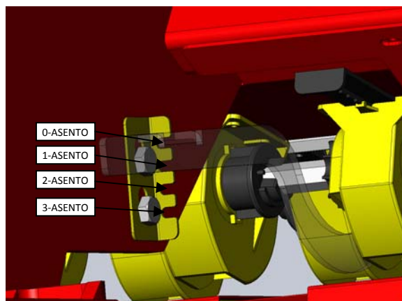
Kuva 3.4.2 Säätövipun loviasteikko.
